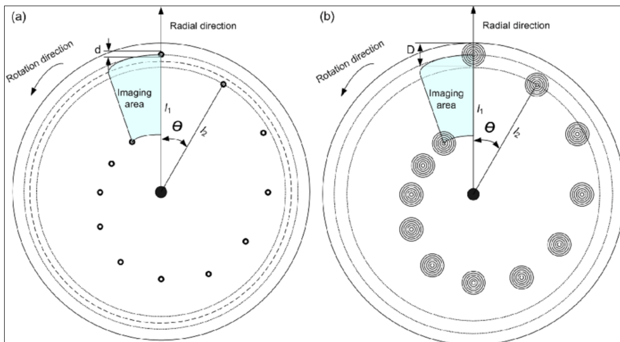
Рисунок 1.1.1 – Ілюстрація диску П. Ніпкова на сайті ResearchGate.
