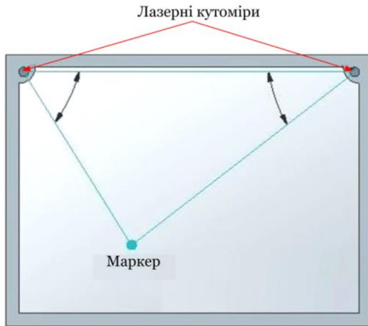
Рис. 2.10. Принцип роботи дошки за лазерною технологією
