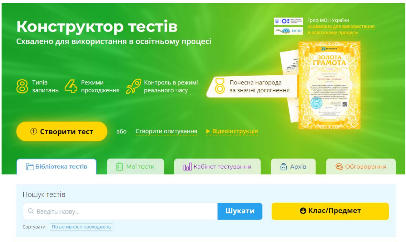
Рис. 3.16. Конструктор тестів
