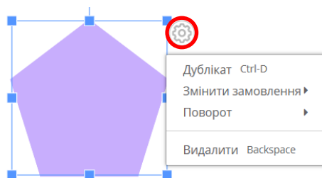
Рис. 2.22. Налаштування об'єкту
