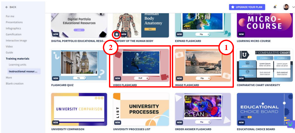
Рис. 2.35. Шаблони флеш-карток
