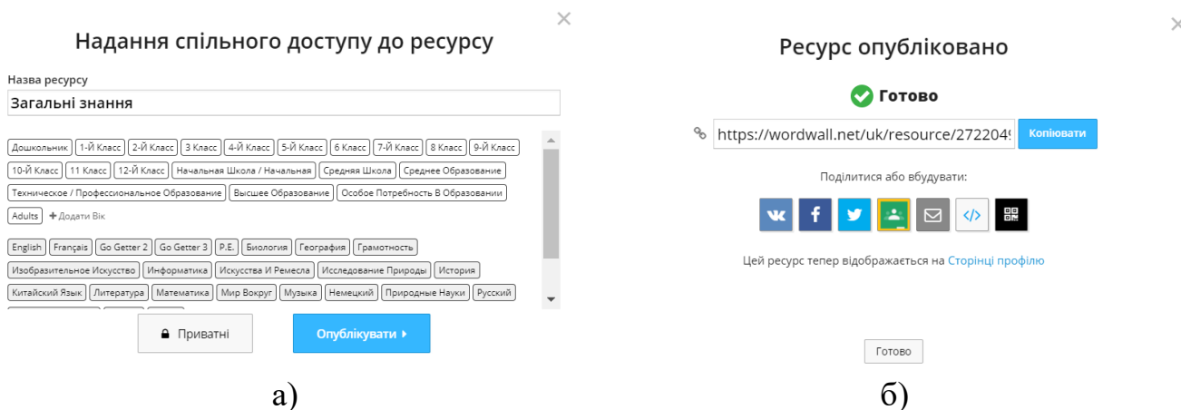
Рис. 3.35. Публікація вправи
