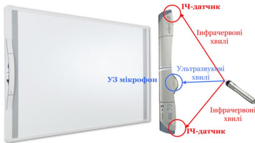
Рис. 2.9. Принцип роботи дошки за інфрачервоною-ультразвуковою технологією
