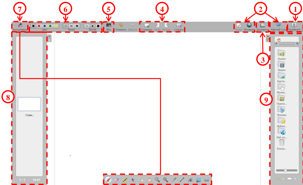
Рис. 2.15. Вікно OpenBoard
