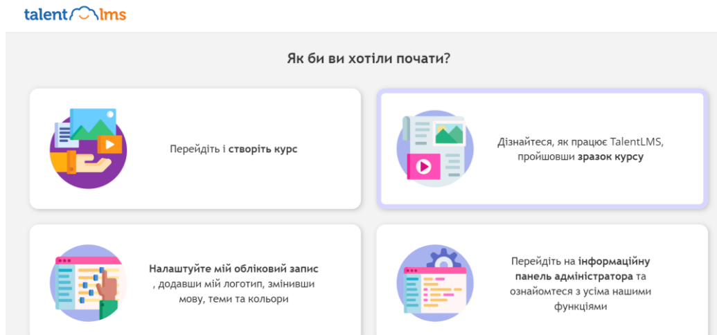
Рис. 5.5. Система TalentLMS
