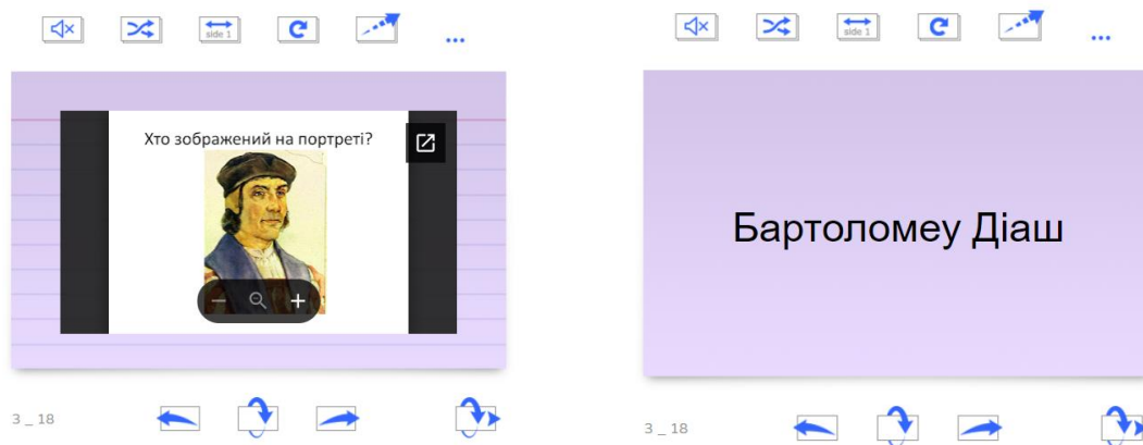
Рис. 2.32. Розроблені флеш-картки
