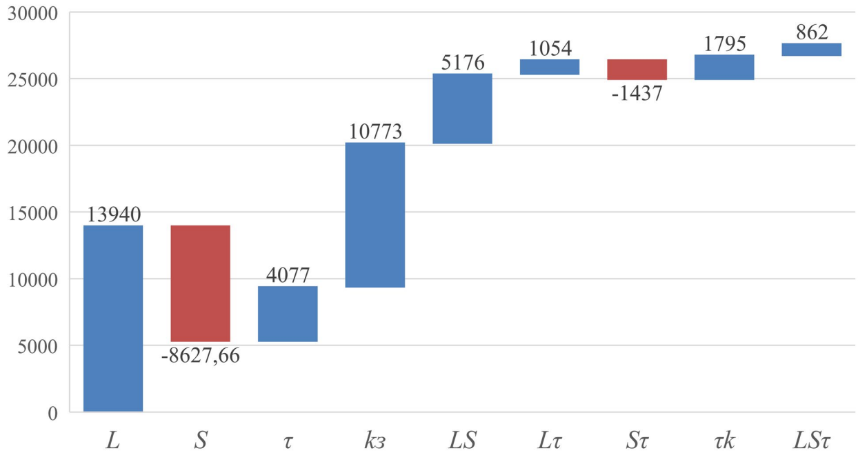
Рисунок 2.3 – Гістограма впливу параметрів на втрату електроенергії
