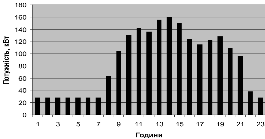
Рисунок 3.2 Добовий графік споживання активної потужності за 12.12.2017р.
