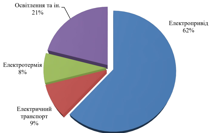
Рисунок 3.1 – Діаграма співвідношення електроенергоспоживання обладнання механічного цеху ТОВ ВКФ «Імпекс»
