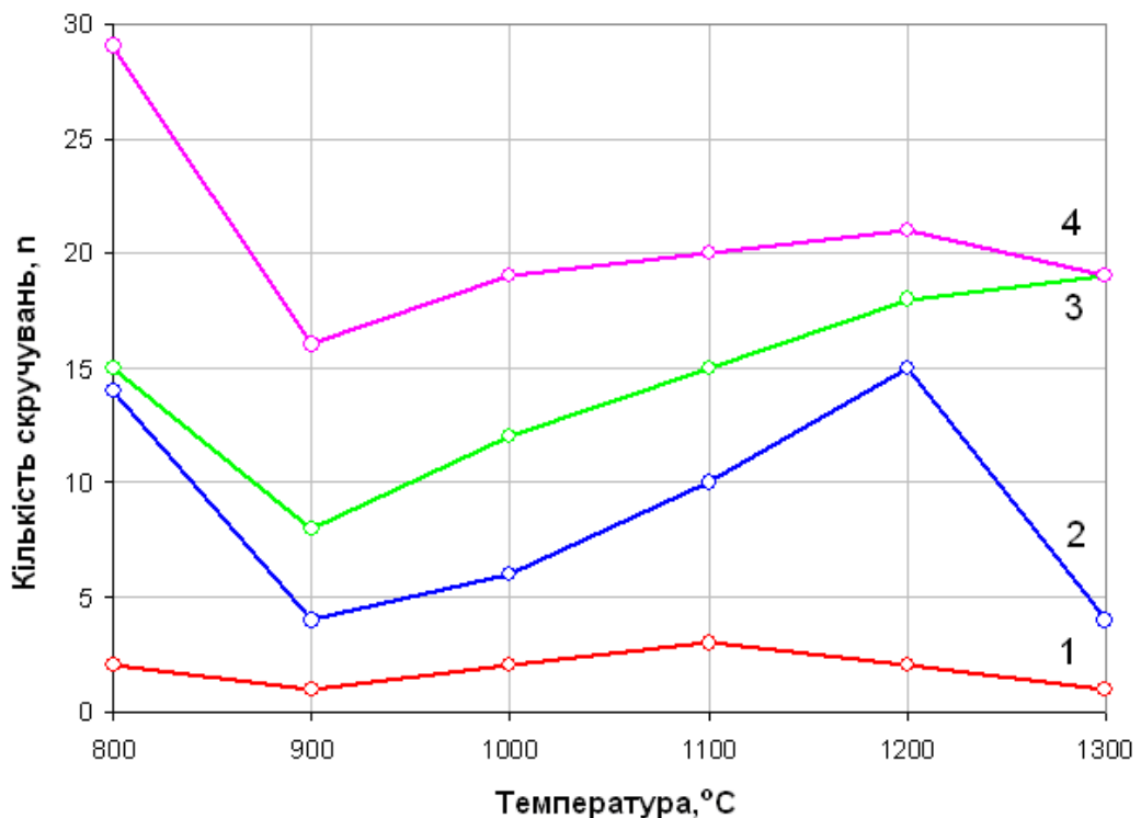
1 - осьова зона зливка масою 1 т; 2 - підповерхнева зона зливку; 3 - периферійна зона зливка; 4 - Периферійна зона заготівлі перетином 180 мм.
