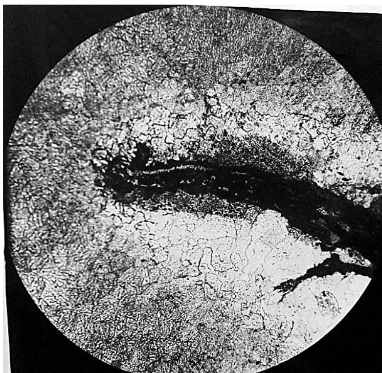
Рисунок 1.5 – Макроструктура металу в місцях дефектів сталі 4X4M2BFC у не відпаленому стані
