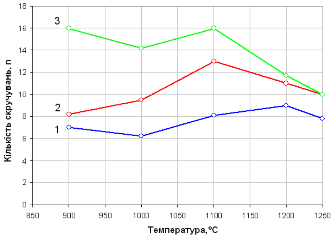
Рисунок 2.3. – Властивості литого (1) та деформованого (2, 3) металу сталі 5X3B3MF при гарячому скручуванні
