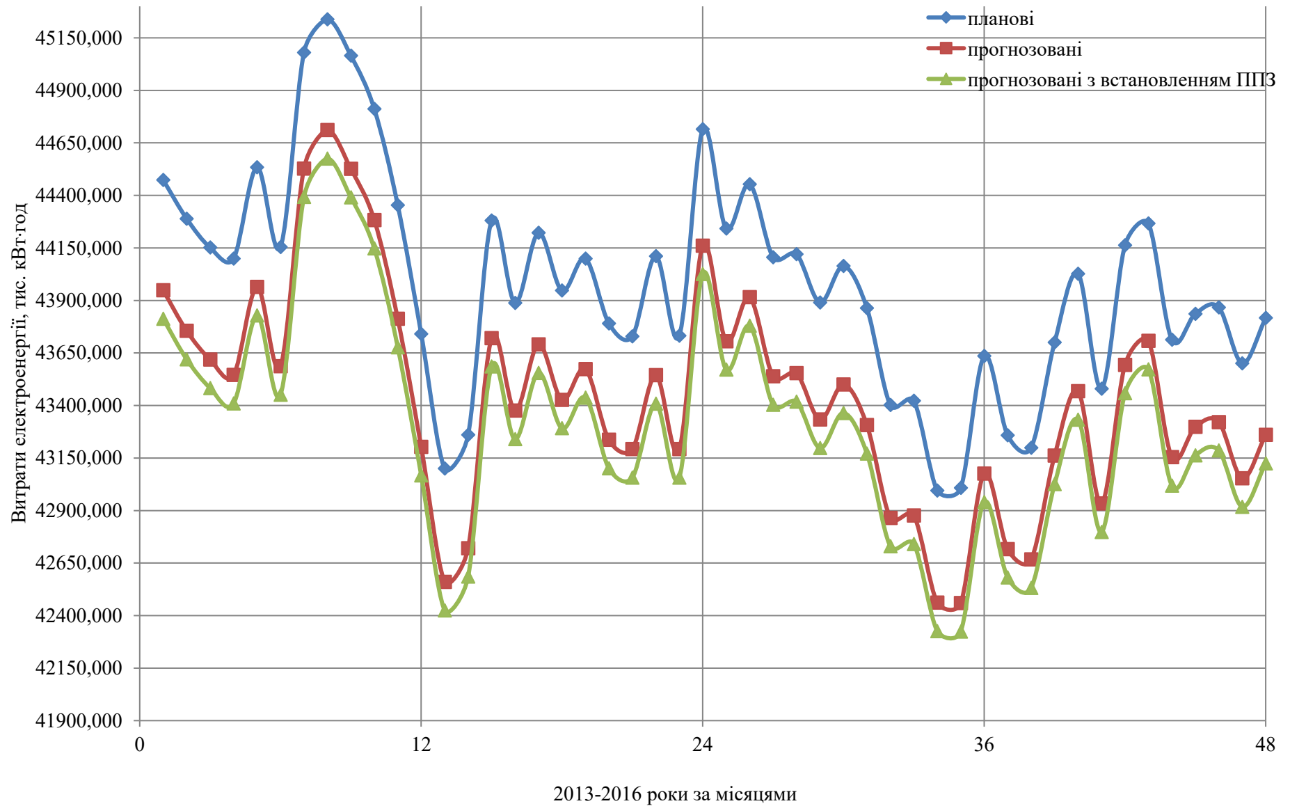
Рисунок 3.1 – Прогнозовані обсяги енергоспоживання киснево-компресорного цеху на 2013–2016 роки
