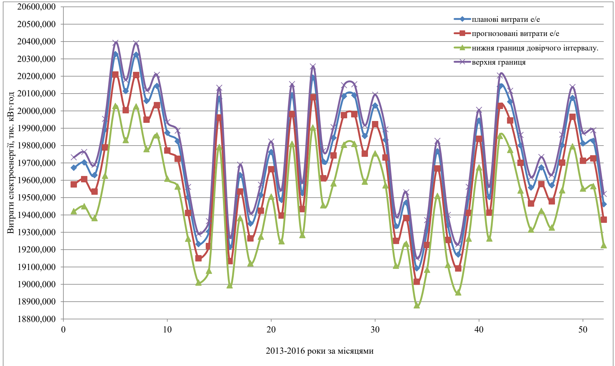
Рисунок 2.5 – Графік електричного навантаження на 2013–2016 роки
