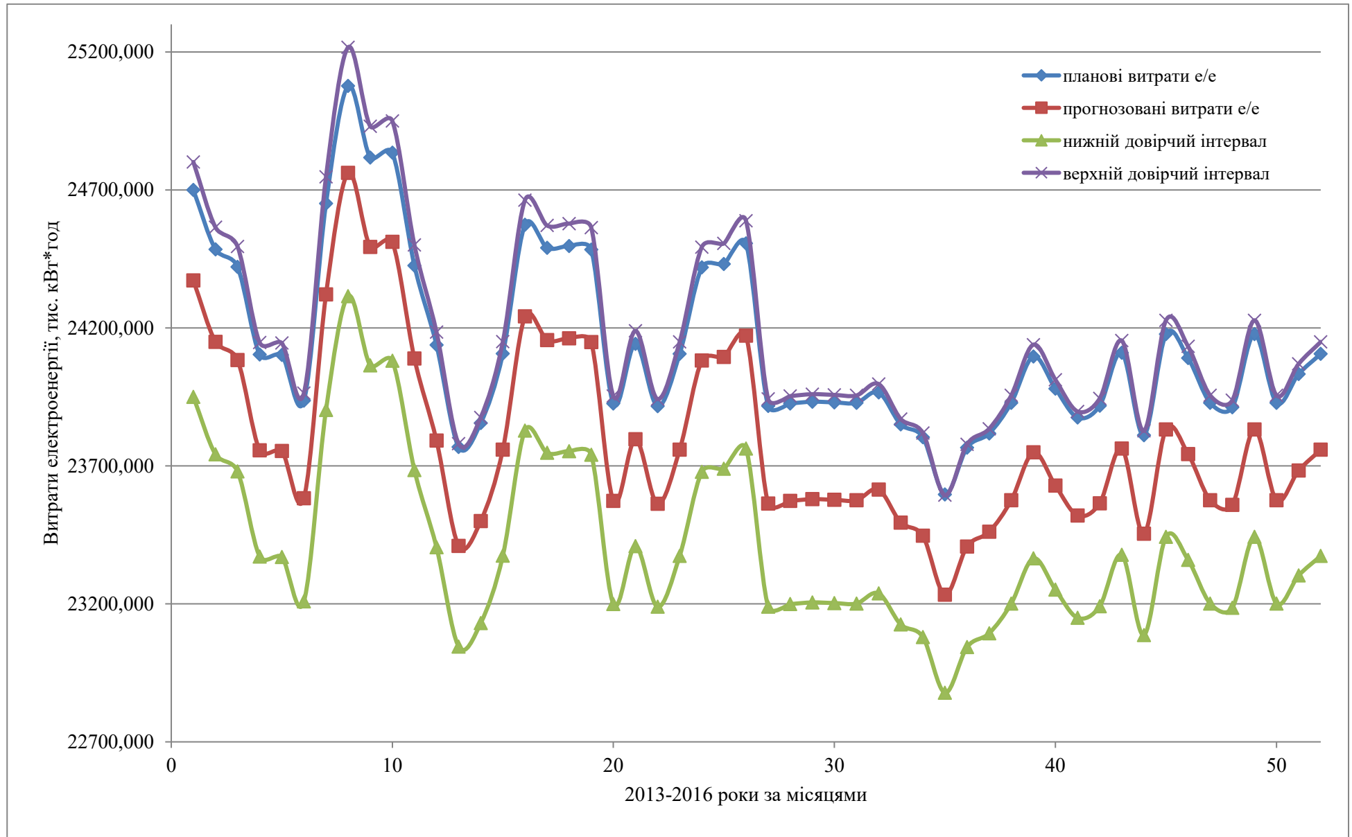
Рисунок 2.2 – Графік електричного навантаження на 2013–2016 роки
