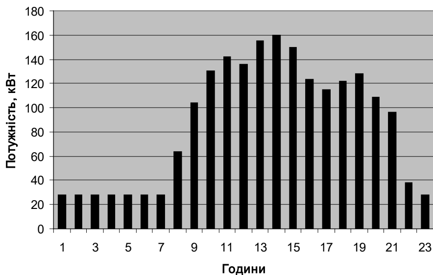
Рисунок 1.4 - Добовий графік споживання активної потужності за 12.12.2022р.
