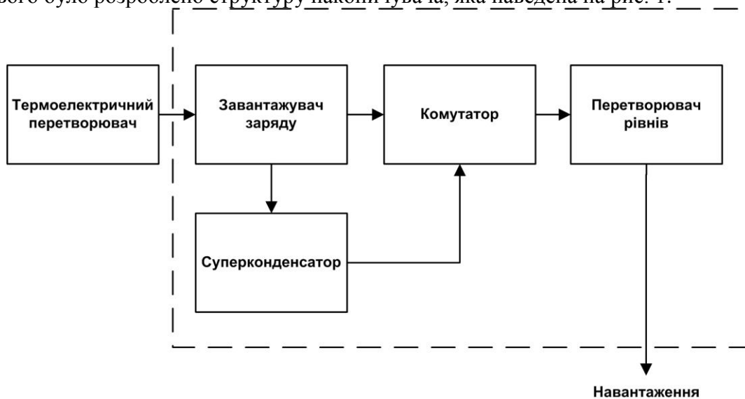
Рисунок 1 – Структура накопичувача електричної енергії
