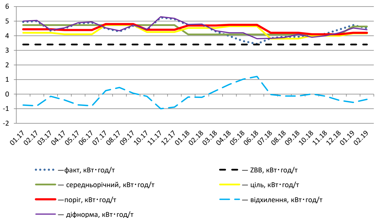
Рисунок 3.1 – Аналіз витрат електроенергії на випуск шихти
