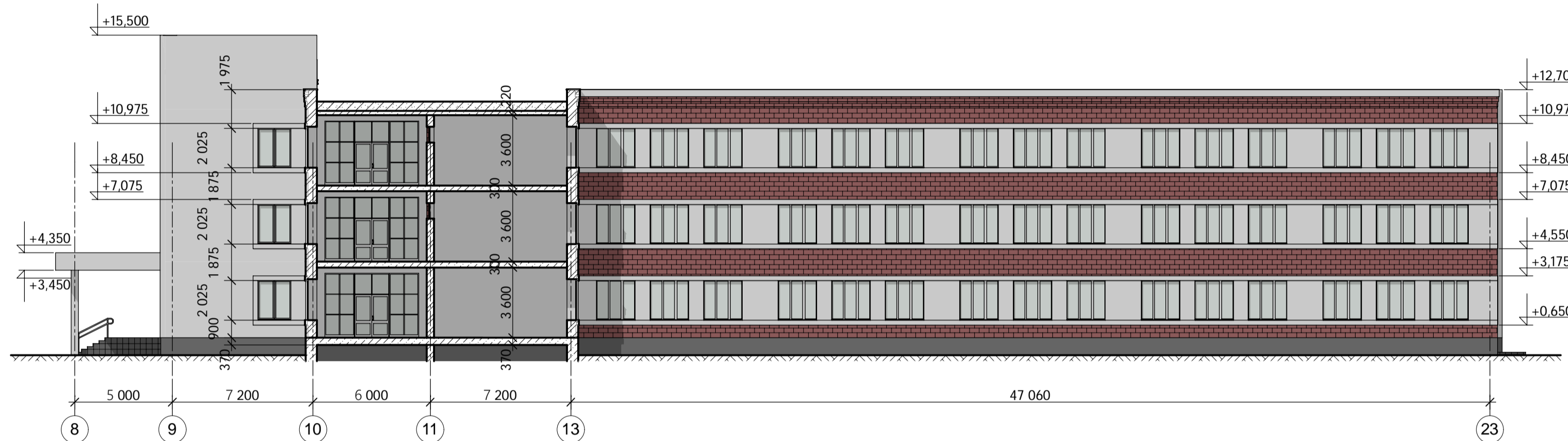
Фрагмент фасаду в осях 9-23 по осі Д
