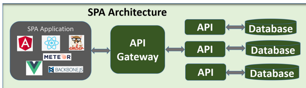
Рисунок 9 — Схема архітектури SPA
