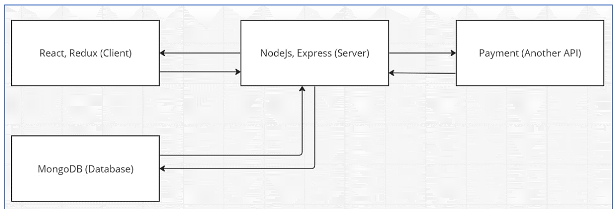
Рисунок 11 — Архітектура системи
