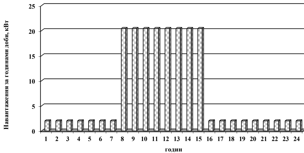
Рисунок 1.5 Добовий графік навантаження освітлювальних установок
