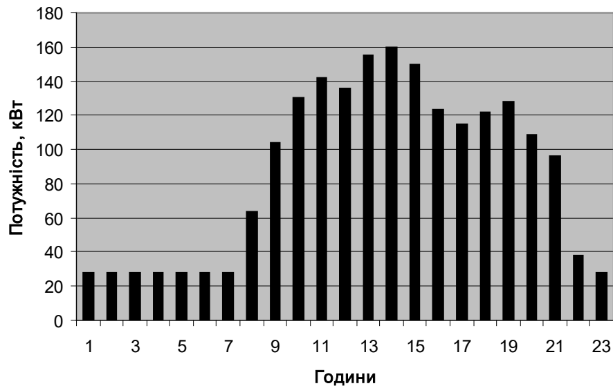
Рисунок 1.4 - Добовий графік споживання активної потужності за 12.12.2023р.
