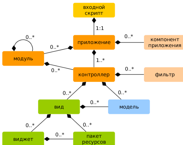
Рисунок 2.2 – Структурна схема MVC
