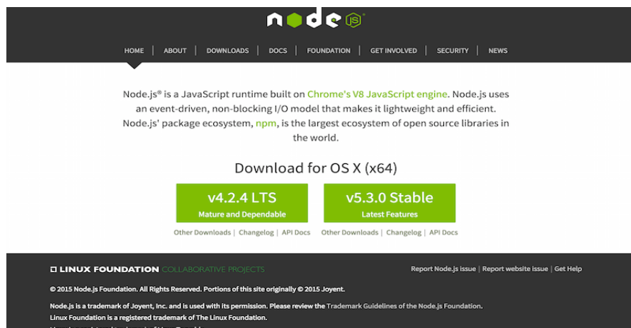
Рисунок 1.2 – Фреймворк Node.js
