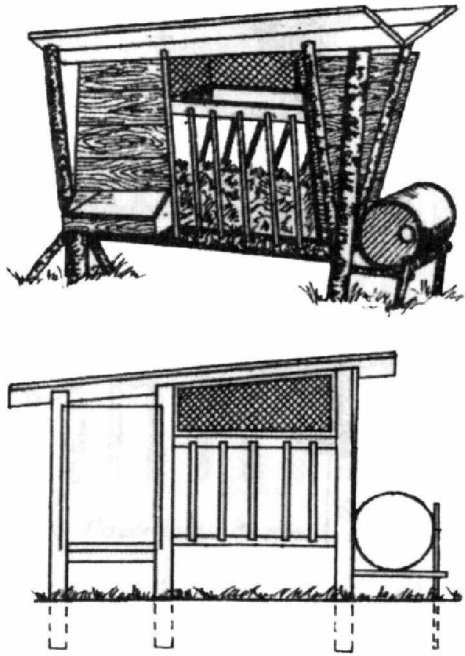
Рис. 6. Універсальна годівниця з бункером для соковитих кормів, яслами для грубих кормів, ящиком для комбікорму та емкістю для сипучих кормів
