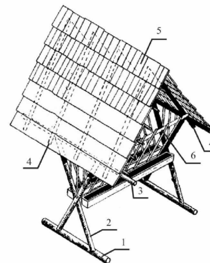
Рис. 2. Складові частини годівниці
