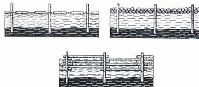
Рис. 6. Хвильоломні присторі
