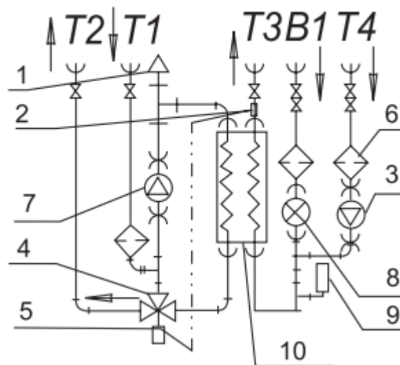
Рисунок 2.6 – Гідралічна схема УГВнс 90
