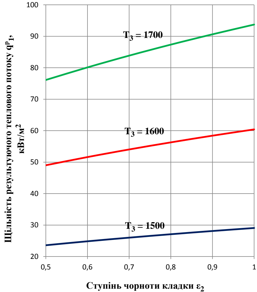
Рисунок 2.8 - Залежність щільності результуючого теплового потоку на метал від ступеня чорноти кладки \epsilon_2 при T_3 = 1400 \text{ K}
