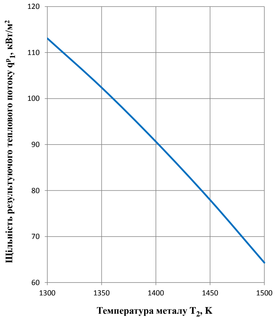
Рисунок 2.14 – Залежність щільності результуючого теплового потоку на метал від температури металу
