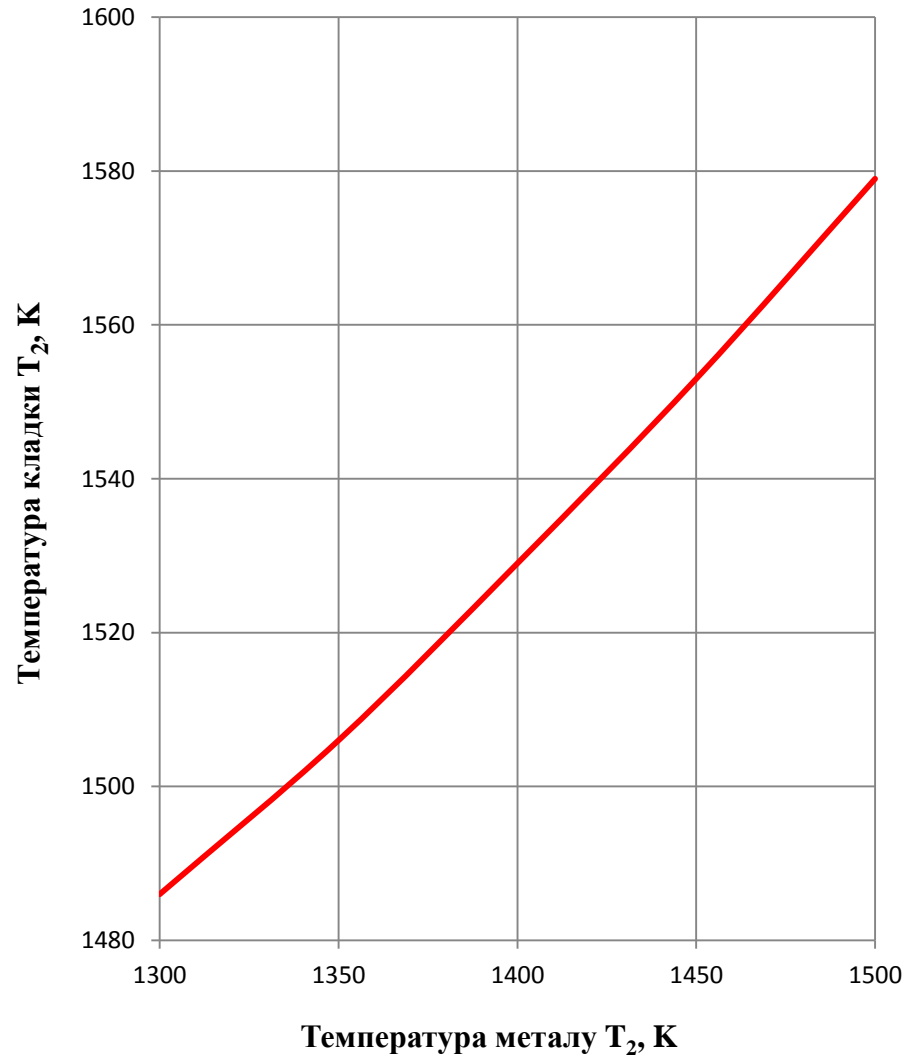
Рисунок 2.13 – Залежність температури кладки T_2 від температури металу
