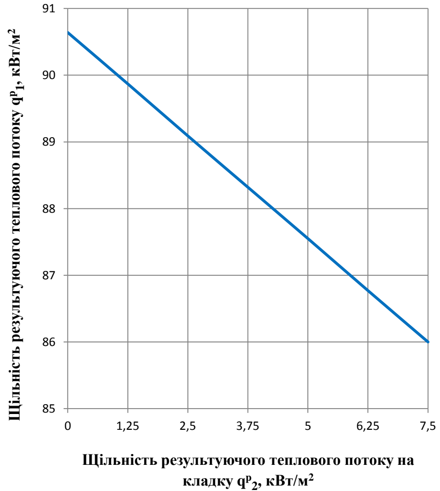
Рисунок 2.16 – Залежність щільності результуючого теплового потоку на метал від щільності результуючого теплового потоку на кладку
