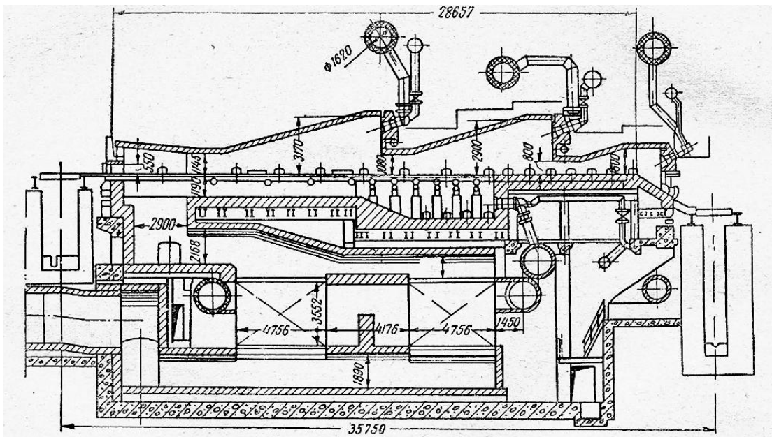
Рисунок 1.8 – Методична нагрівальна піч зі здвоєної зварювальної зоної
