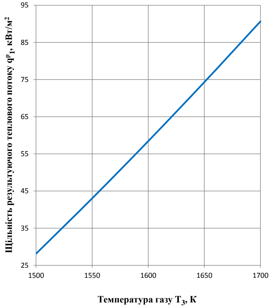
Рисунок 2.10 – Залежність щільності результуючого теплового потоку на метал від температури газу
