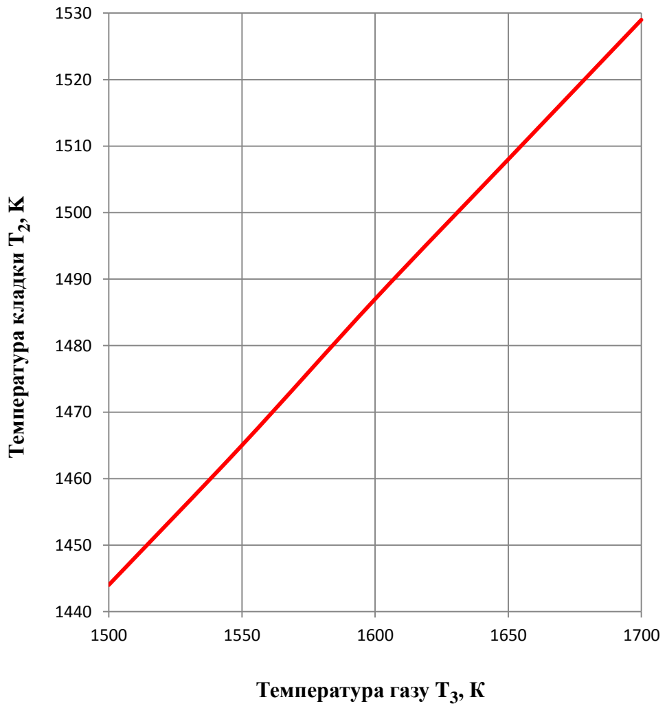
Рисунок 2.9 – Залежність температури кладки від температури газу
