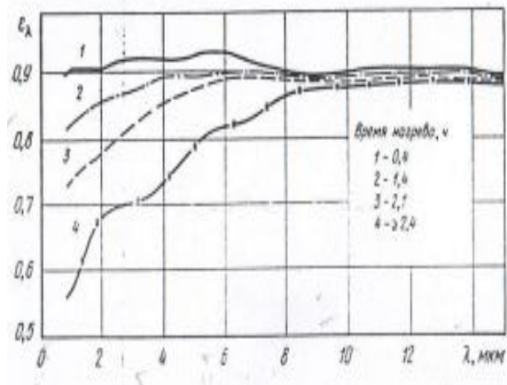
Рисунок 1.4 - Залежність спектральної ступеня чорноти окалини від довжини хвилі при різному часі нагріву металу в методичній печі
