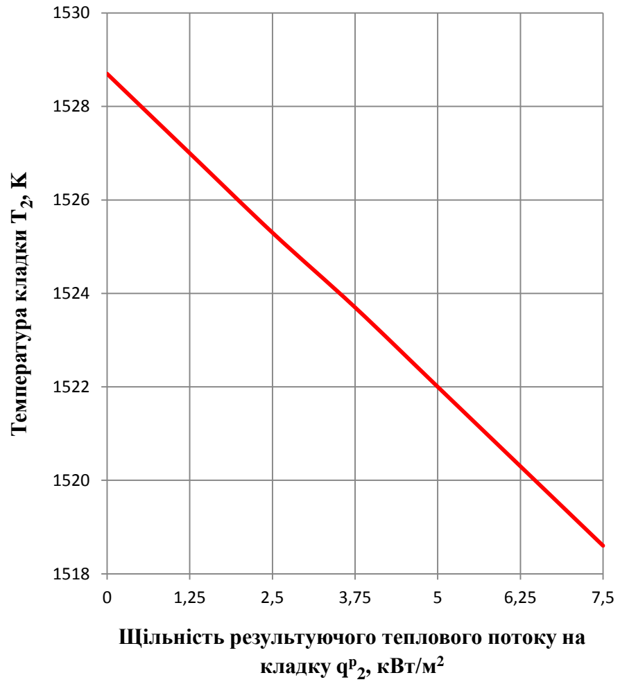
Рисунок 2.15 – Залежність температури кладки T_2 від щільності результуючого теплового потоку на кладку
