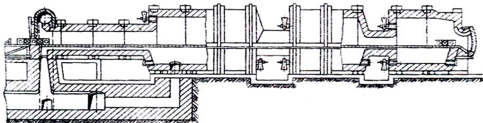
Рисунок 1.9 – Тризонна методична піч з інтенсивною циркуляцією газів в герметизованому робочому просторі
