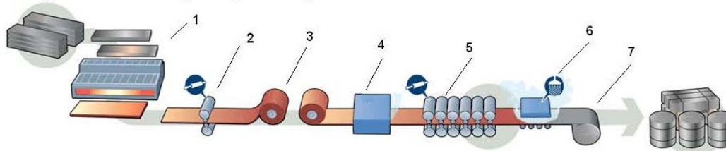
1 - нагрівальні печі; 2 - група чорнових клітей; 3 - проміжний накопичувач Coilbox; 4 - зварювальна установка; 5 - група чистових клітей; 6 - ділянка охолодження на виході; 7 - моталки
