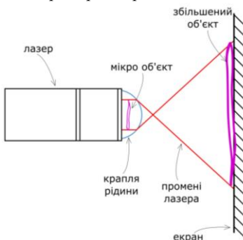
Рисунок 1 – Схема тіньового мікроскопу
