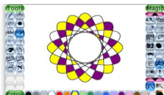
Рисунок 3 – Середовище Omnitux
