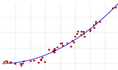
Рисунок 2 – Приклад функції апроксимації дискретного набору точок
