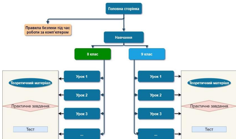
Рисунок 1 – Схема вебресурсу
