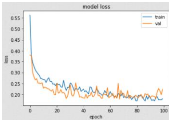
Рисунок 1 – Зображення функції помилки
