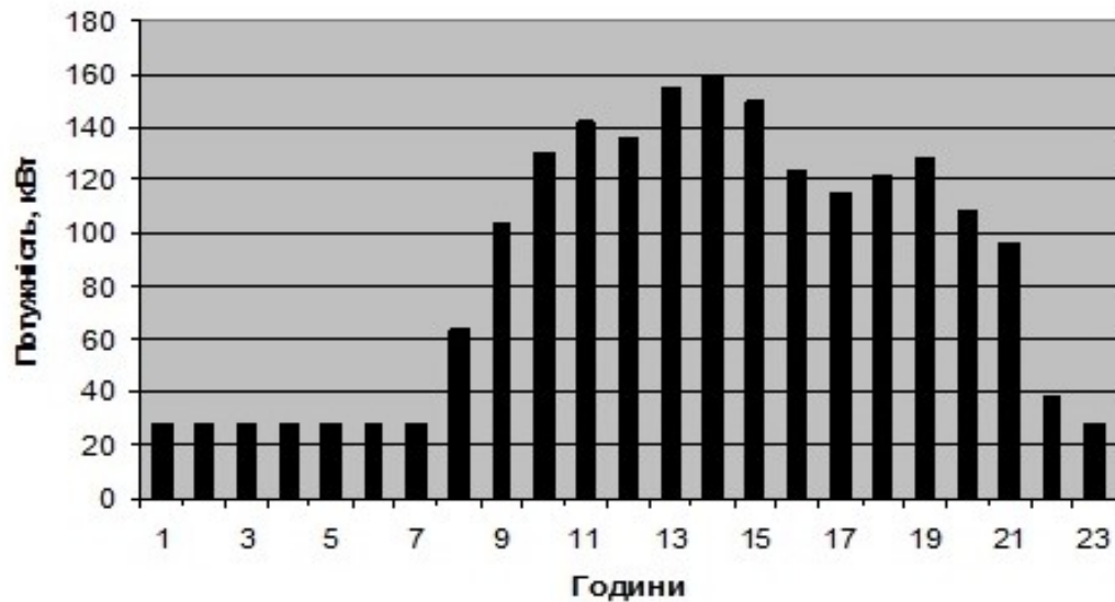
Рисунок 2.1 Добовий графік споживання активної потужності за 12.12.2021р.
