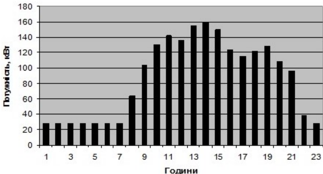
Рисунок 1.4 - Добовий графік споживання активної потужності за 12.12.2021р.
