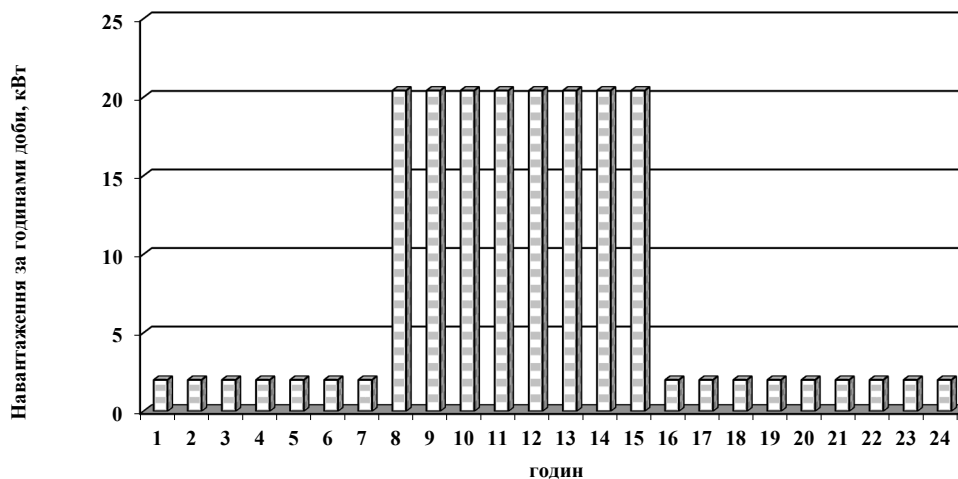
Рисунок 1.7 Добовий графік навантаження освітлювальних установок
